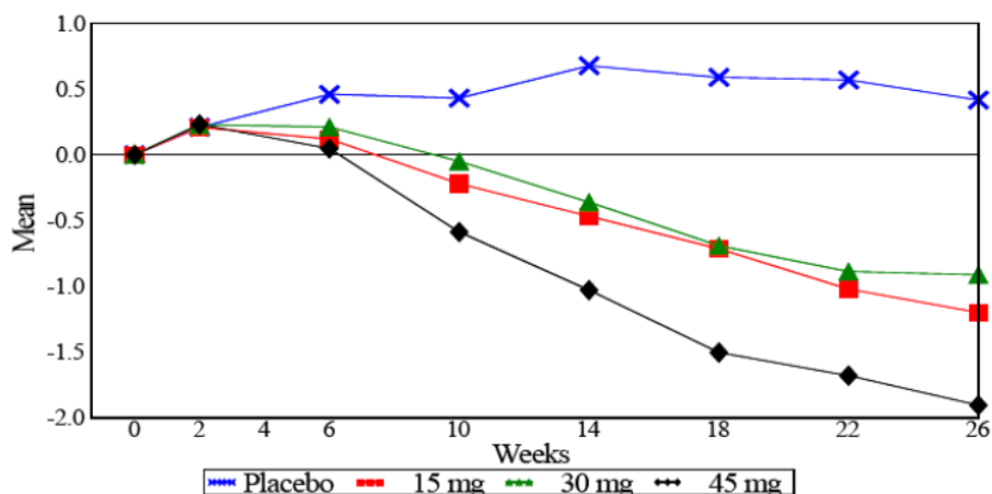
Figura 1: Alteração média do valor basal para HbA1c em um estudo de variação de dose placebo-controlado de 26 semanas (valores observados) – Estudo PNFP-001
