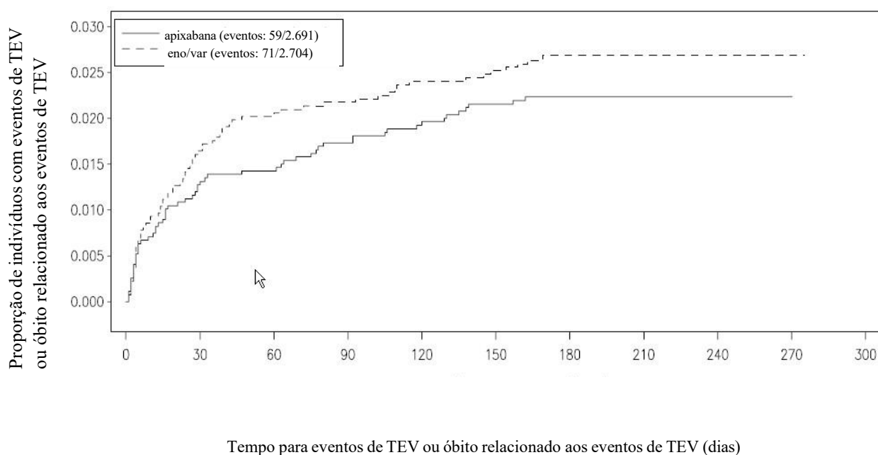
Figura 5: Estimativa de tempo de Kaplan-Meier até a primeira TVP ou EP, ou óbito relacionado aos eventos de TEV no estudo AMPLIFY (população com intenção de tratar)
