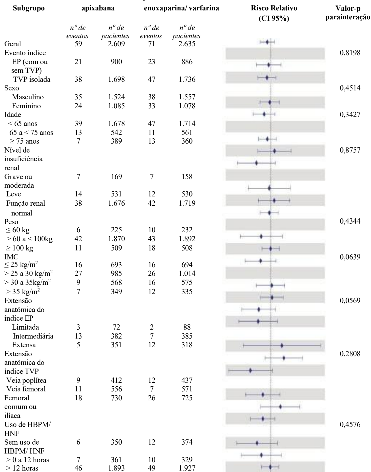
Figura 6: Eventos de TEV sintomático recorrente (TVP não fatal ou EP não fatal) ou risco relativo de óbito relacionado aos eventos de TEV pelas características basais:
