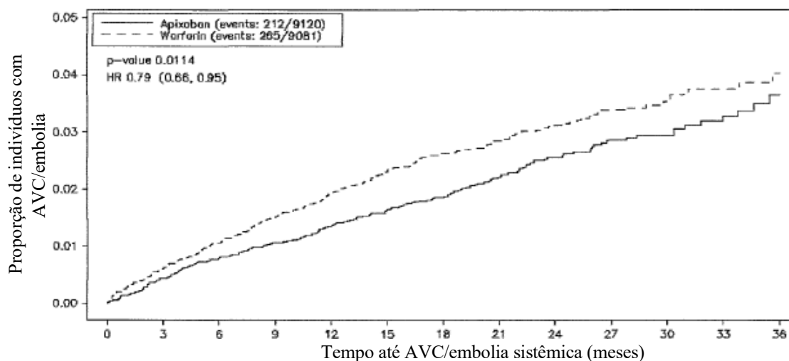
Figura 1: Estimativa da curva de Kaplan-Meier de tempo para a ocorrência do primeiro AVC ou embolia sistêmica no estudo ARISTOTLE
