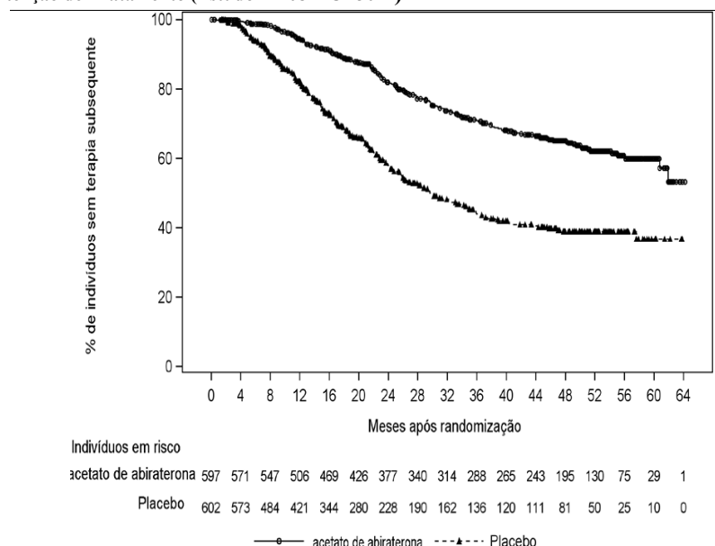
Figura 3: Gráfico de tempo até a terapia subsequente que prolonga a vida para o câncer de próstata de Kaplan-Meier; População com Intenção de Tratamento (Estudo 212082PCR3011)
